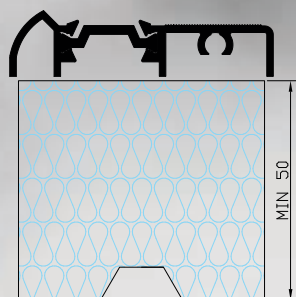
EXSP-800 THRESHOLD EXTENSION ΠΡΟΕΚΤΑΣΗ ΚΑΤΩΚΑΣΙΟΥ
