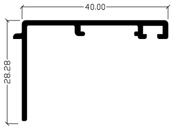
EXSP-802 INTERNAL COVERING ΕΣΩΤΕΡΙΚΟ ΠΕΡΒΑΖΙ
