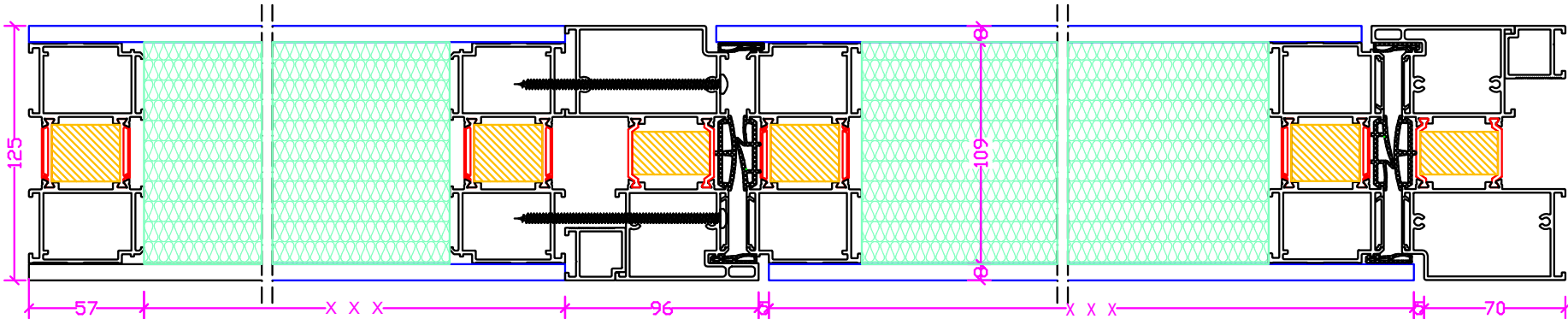
ΤΟΜΗ A-A / SECTION A-A
