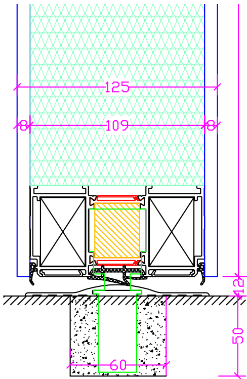
ΜΟΝΟΦΥΛΛΗ ΠΟΡΤΑ ΜΕ ΦΕΓΓΙΤΗ SINGLE LEAF DOOR WITH TOP PART
