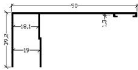
EXSP-803 EXTERNAL COVERING ΕΞΩΤΕΡΙΚΟ ΠΕΡΒΑΖΙ
